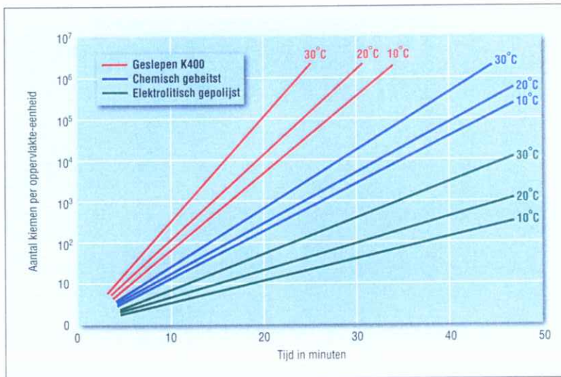
Afbeelding 4: Duidelijk is het effect te zien van elektrolytisch gepolijst oppervlak m.b.t. de afzet van vreemde deeltjes. (Bron: Packo België)
