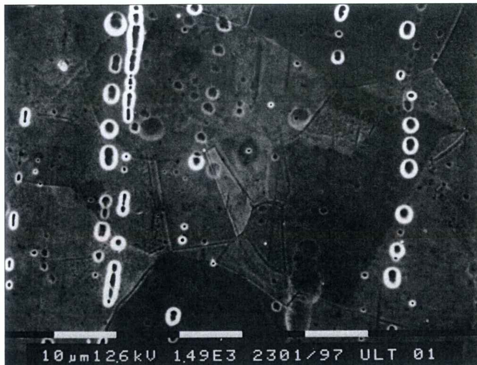
Afbeelding 2: Elektrolytisch gepolijst roestvast staal 316L oppervlak dat geen kanaalvorming meer toont op de korrelgrenzen. V = 1500\times . (Foto: Dockweiler Nederland)
