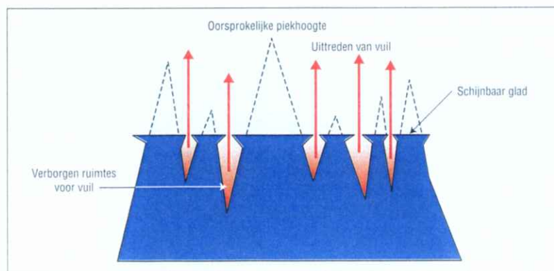
Afbeelding 3: Schematische voorstelling op microschaal. Mechanisch polijsten drukt ook de toppen enigszins dicht waardoor vuil zich op kan hopen. Bij een thermische uitzetting komt het vuil naar buiten en/of naar binnen.
