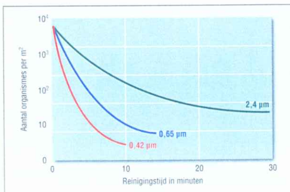
Afbeelding 5: De reinigingstijd als functie van de ruwheid van het roestvast staal oppervlak. (Bron: Packo België)
